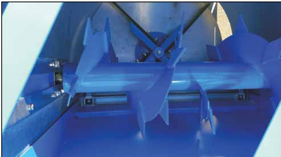
Schnecke zur Zerkleinerung und horizontale Auswurfflügel
